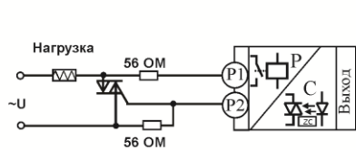
Подключение внешнего симистора
