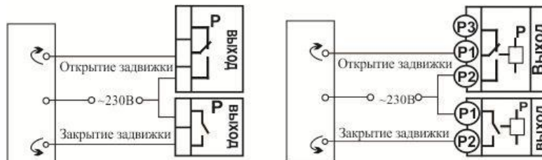
Подключение электрозадвижки
