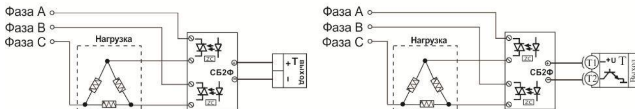
Использование двухфазных силовых блоков для управления трехфазной нагрузкой. Схема подключения «Треугольник»
