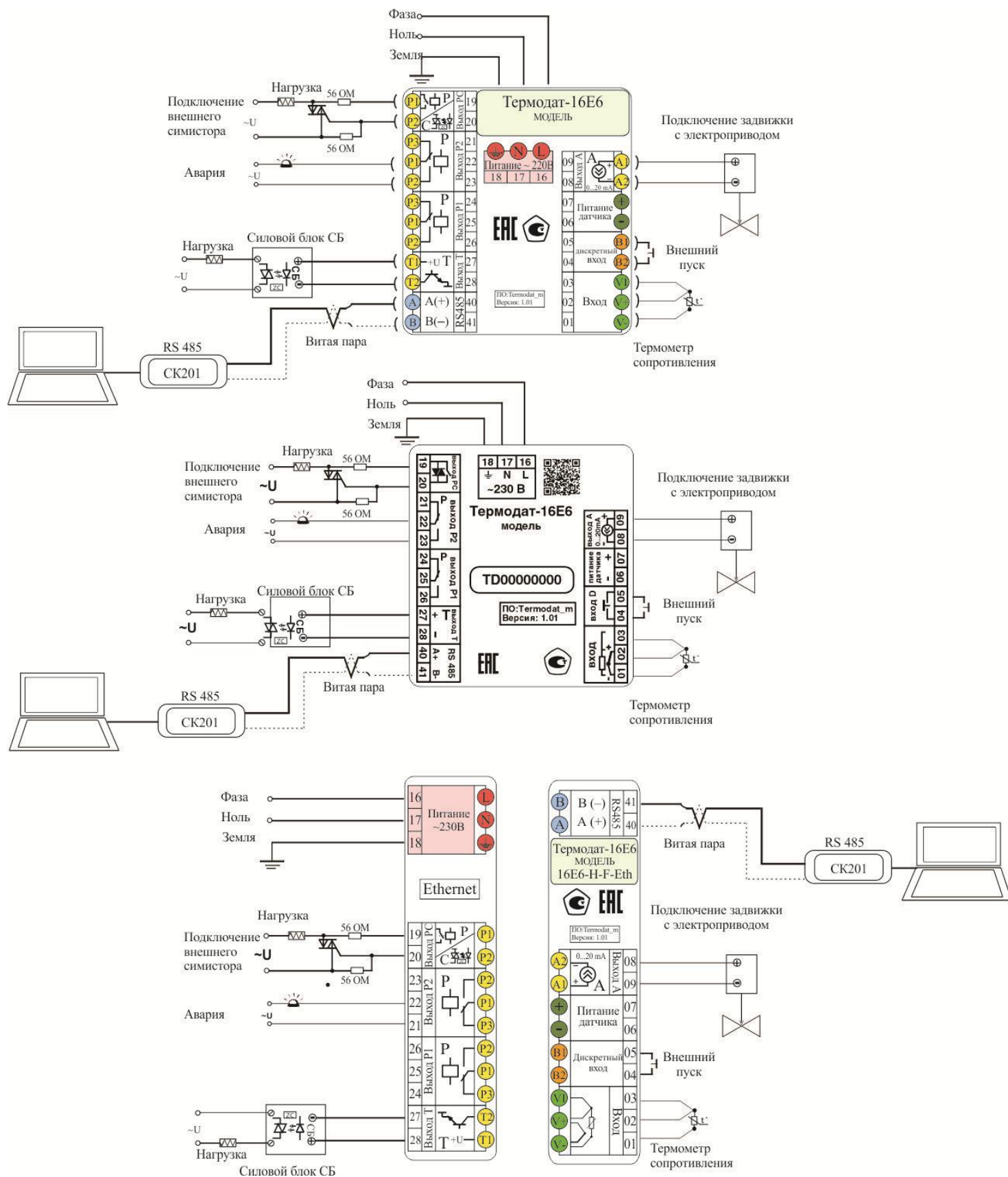
Рисунок 12 – Схема подключения прибора
