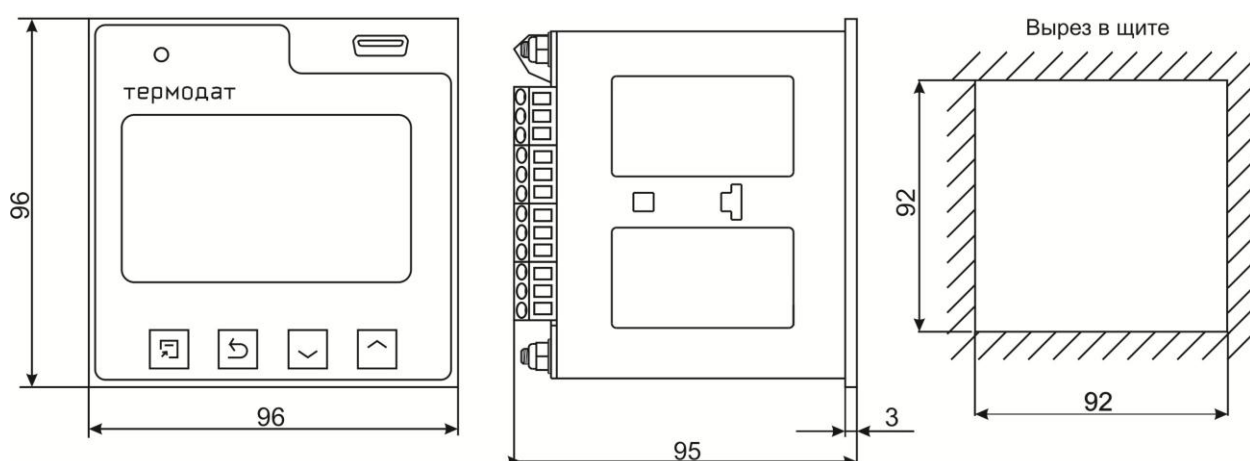
Рисунок 13 – Габаритные размеры прибора Термодат-16Е6/...../(F) или Термодат-16Е6-А-(F)-(Eth)
