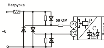
Подключение внешних тириستоров
