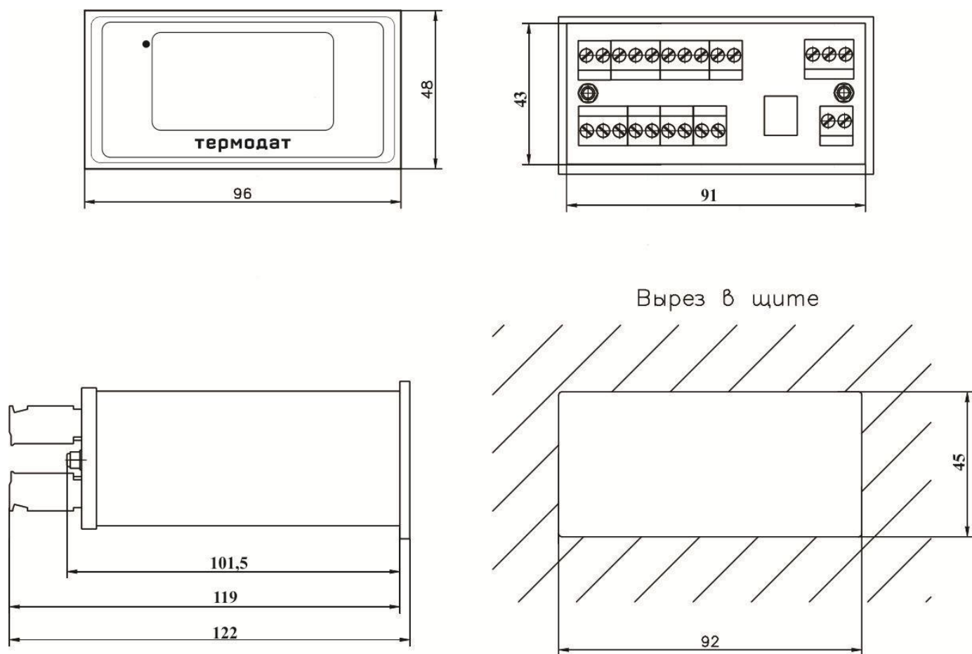
Рисунок 16 – Габаритные размеры прибора Термодат-16E6-D8/..... или Термодат-16E6-H-(F)-(Eth)
