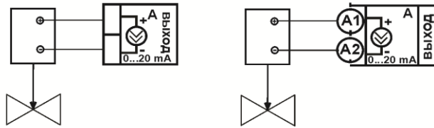
Подключение задвижки с электроприводом
