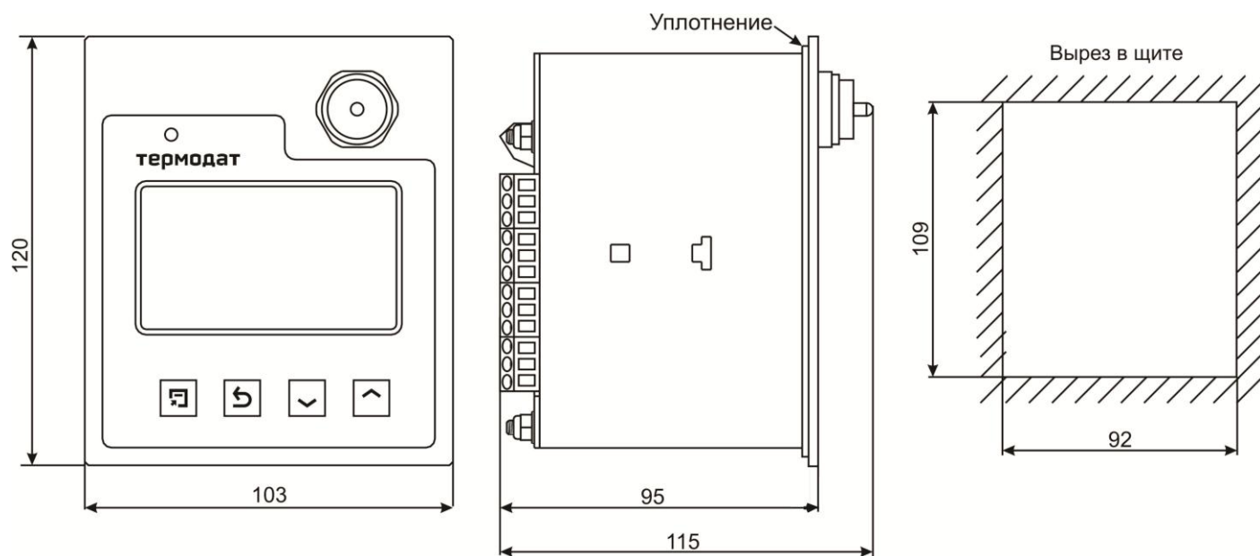
Рисунок 14 – Габаритные размеры прибора Термодат-16Е6/...../IP67пп или Термодат-16Е6-А7
